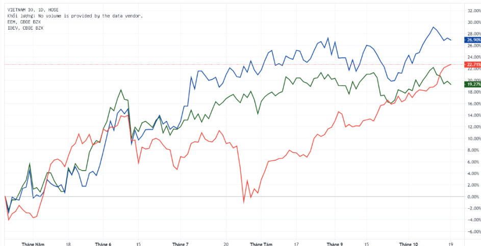
Biểu đồ tương quan biến động VN30 đối với Thị trường phát triển và Thị trường mới nổi 21/10/2020
